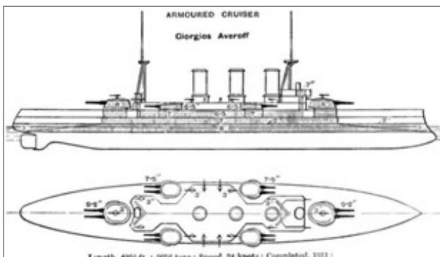
Ill. 8 - Plantegning af "Georgios Averof"
